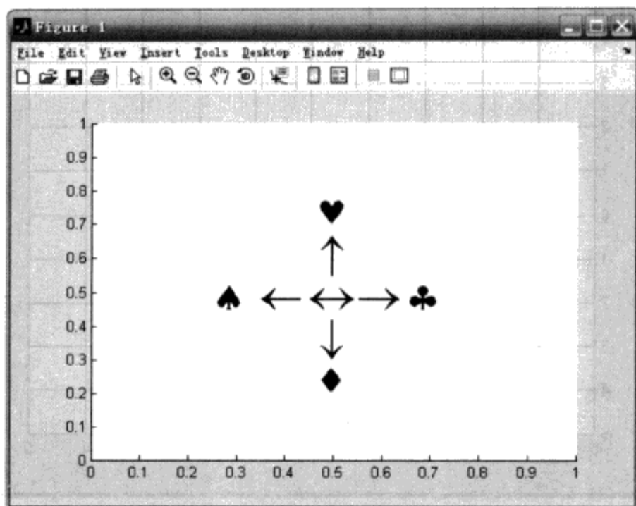
图 3.33 例 3.3.3 图
