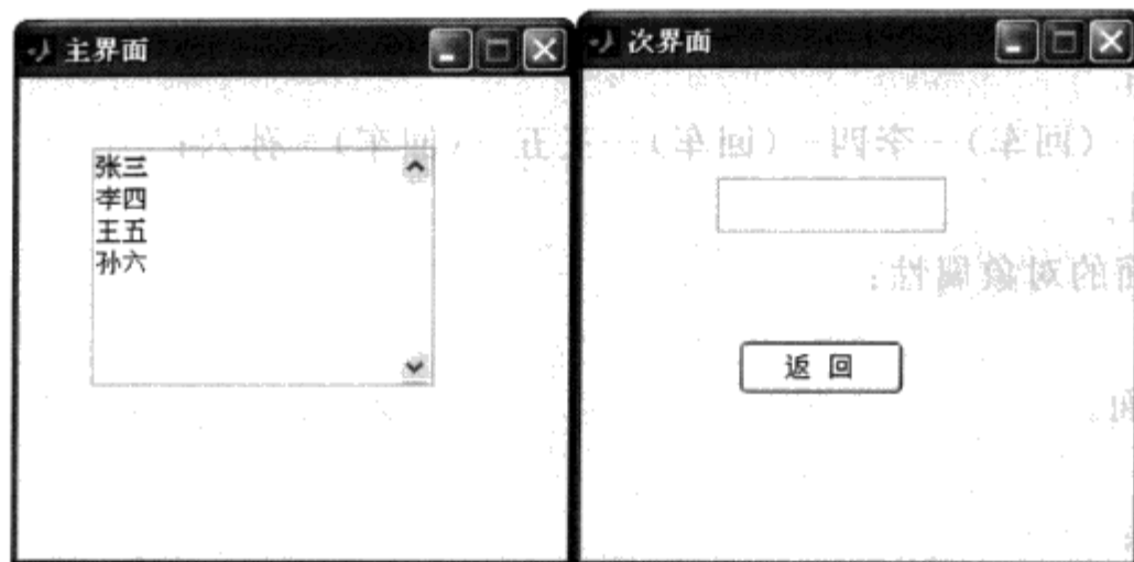
图 6.52 例 6.3.1 图
