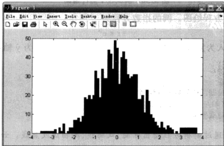
图 3.32 例 3.3.2 运行结果
