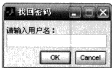
图 5.31 输入对话框
