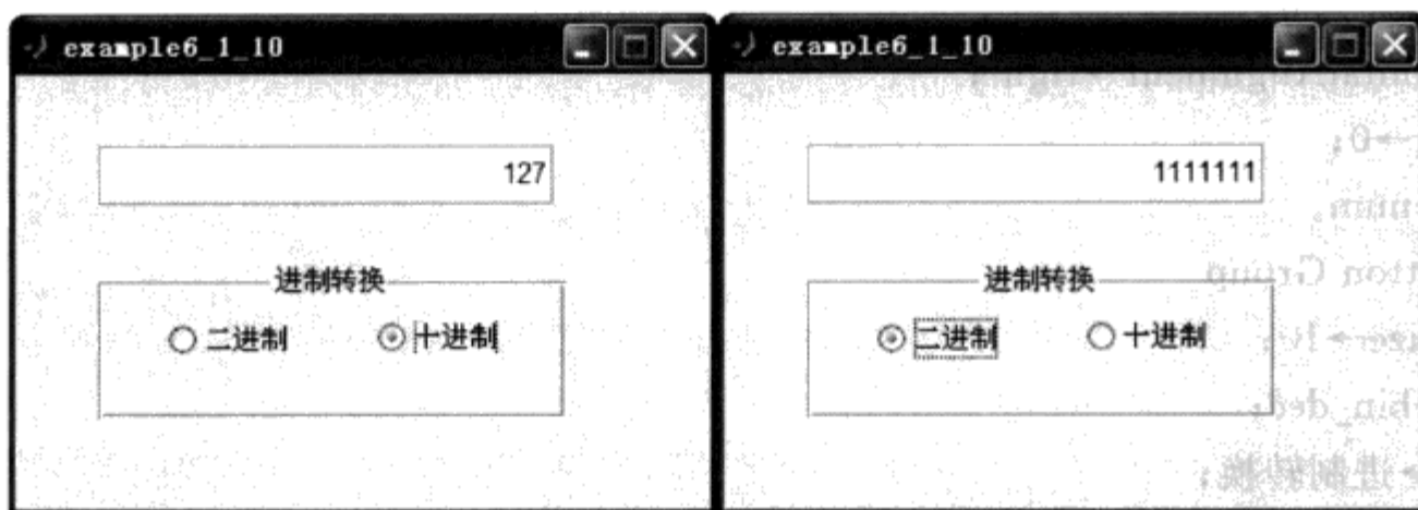
图 6.45 例 6.1.10 运行结果
