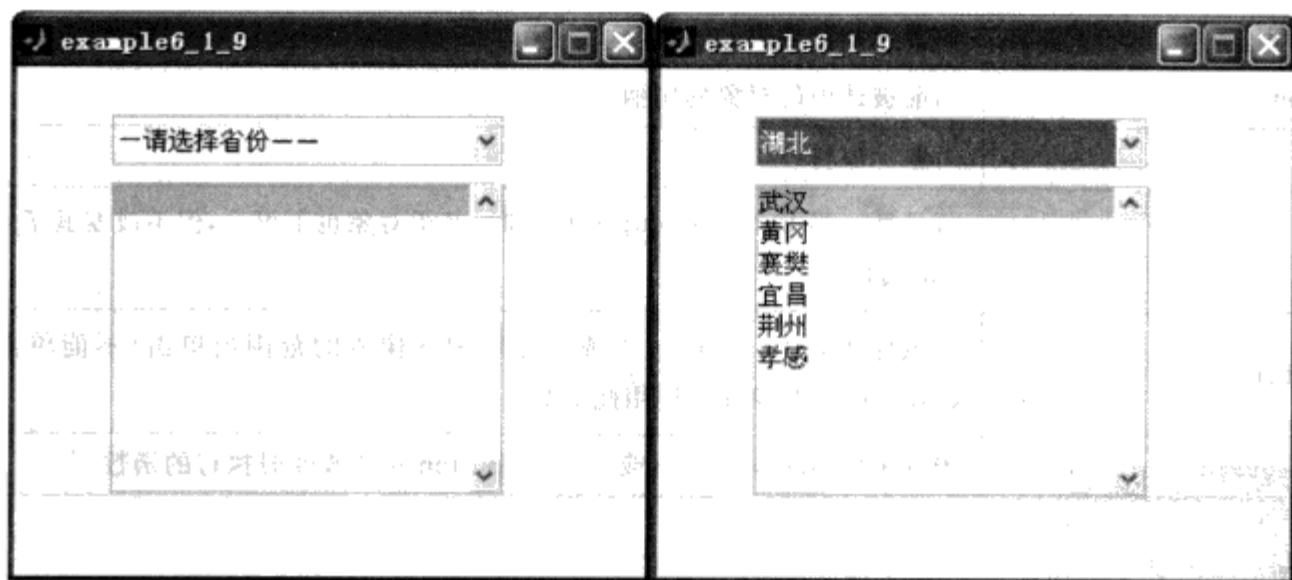
图 6.44 例 6.1.9 运行结果
