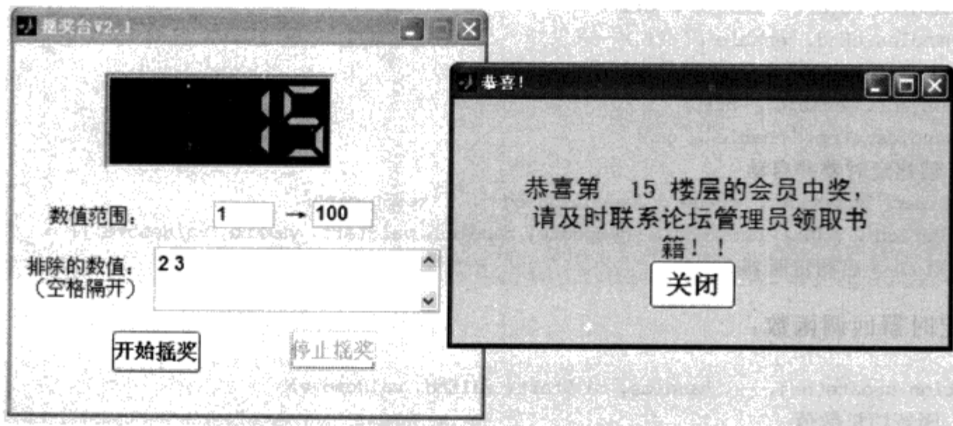
图 8.6 例 8.3.3 运行结果
