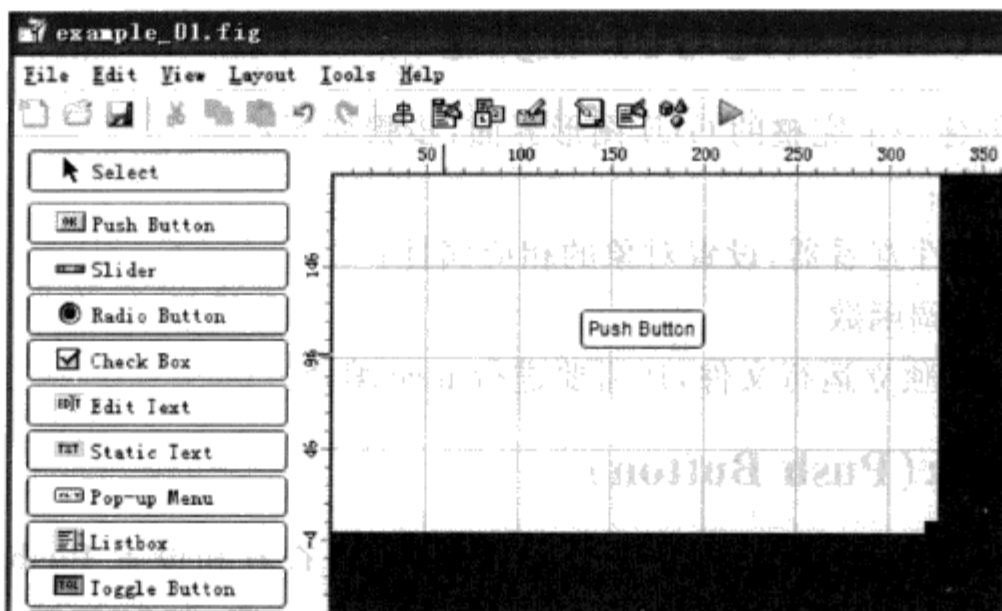
图 6.26 GUI 布局
