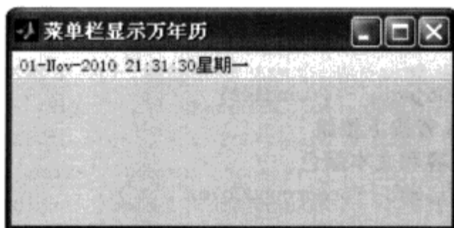
图 8.8 例 8.4.2 运行结果
