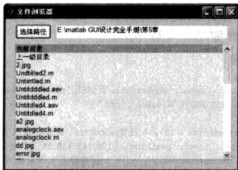
图 5.42 例 5.3.3 运行结果
