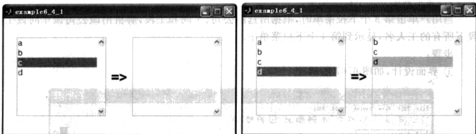
图 6.65 例 6.4.1 运行结果
