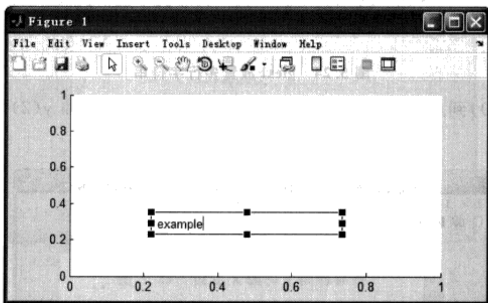
图 3.26 文本注释框
