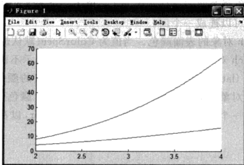
图 4.28 例 4.1.1 原图
