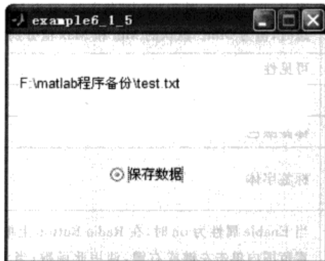
图 6.39 例 6.1.5 运行结果
