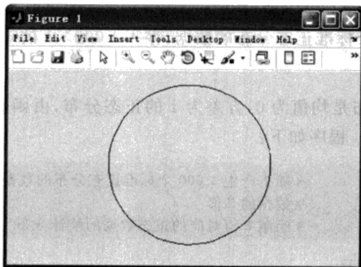
图 3.30 例 3.3.1 运行结果
