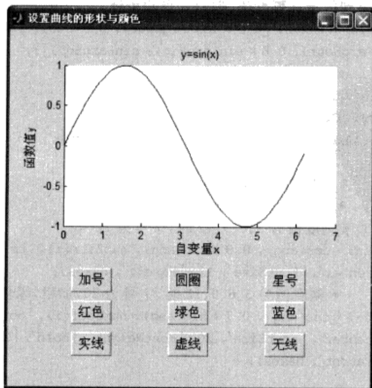
图 4.87 例 4.4.1 原图
