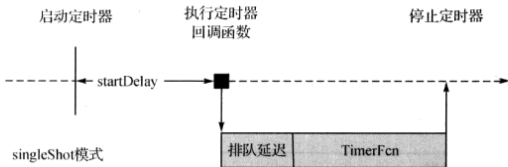
图 8.1 singleShot 模式
