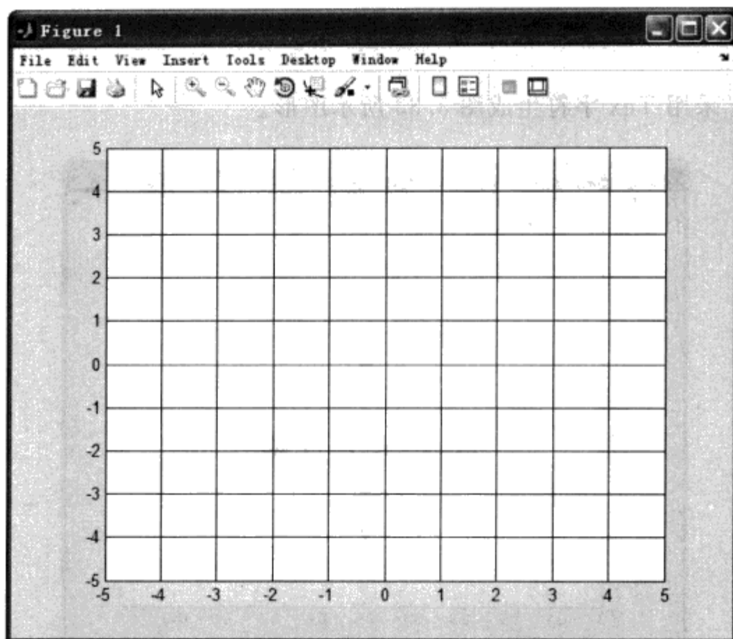
图 3.34 例 3.3.4 网格图
