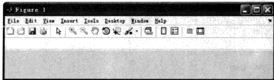
图 4.46 创建工具栏
