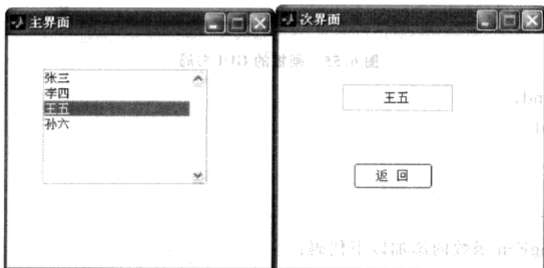
图 6.54 例 6.3.1 运行结果
