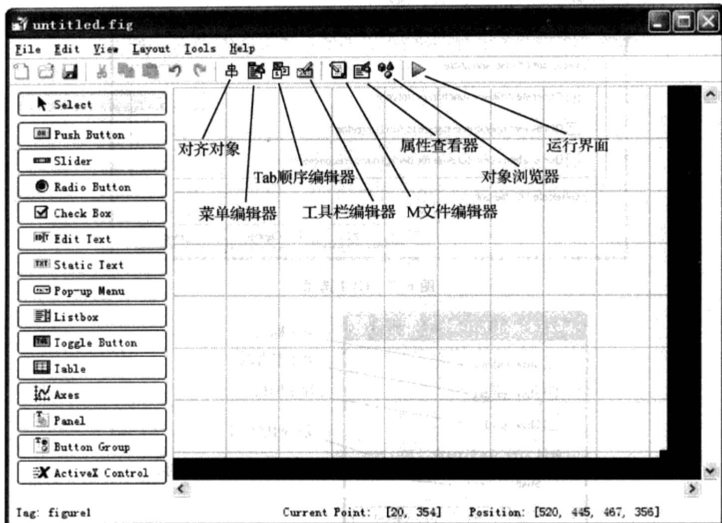
图 6.5 GUI 工具栏
