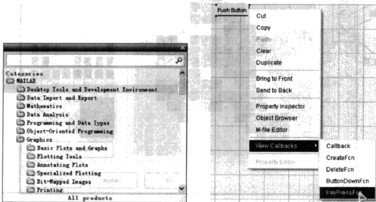
图 6.16 函数浏览器
