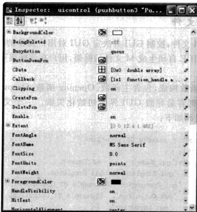
图 6.20 属性查看器
