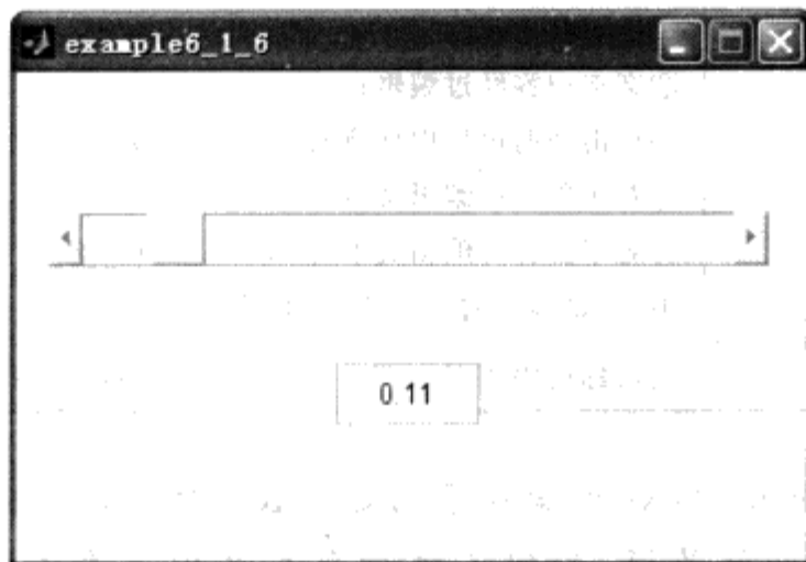
图 6.40 例 6.1.6 运行结果
