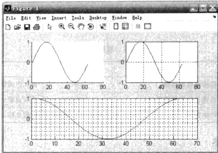
图 3.13 例 3.1.2 运行结果
