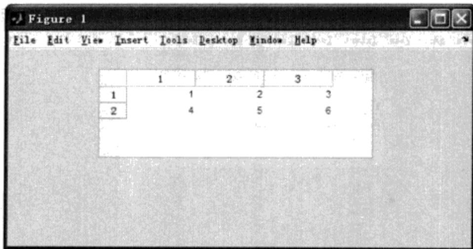
图 4.59 创建表格
