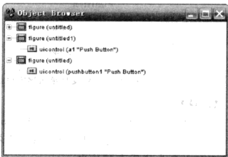
图 6.21 对象浏览器
