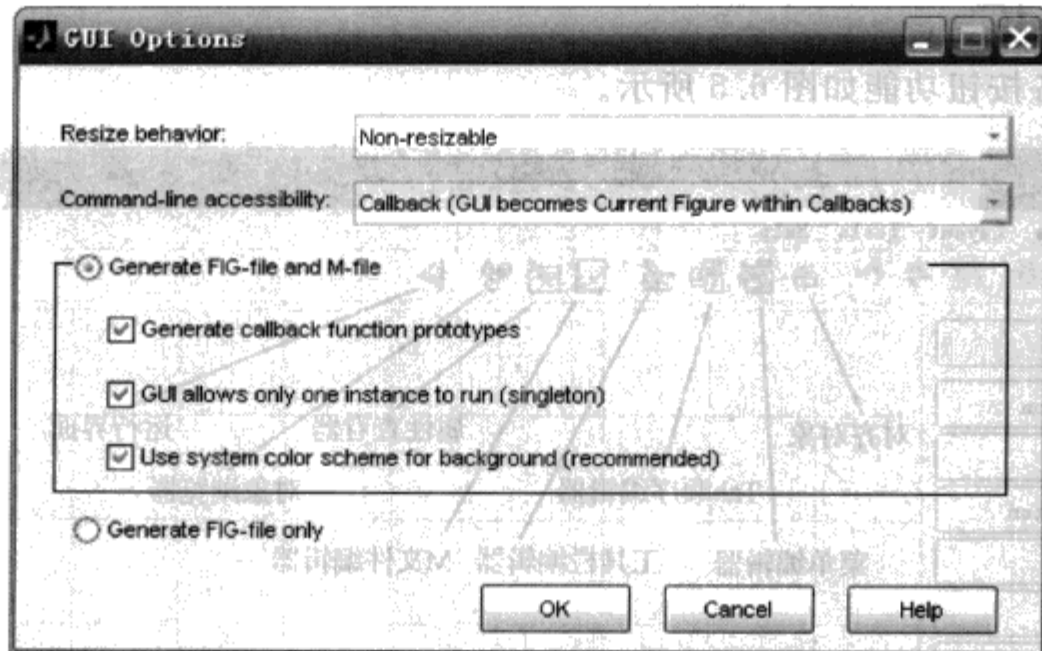
图 6.7 GUI 选项
