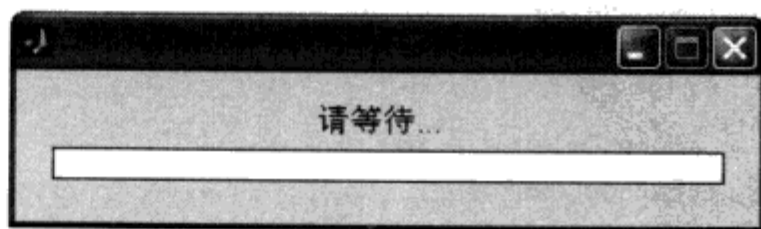
图 5.11 进度条
