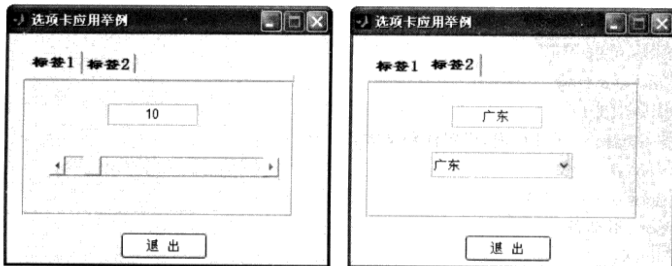
图 7.42 例 7.3.1 运行结果
