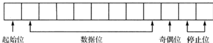
图 9.5 串口数据格式
