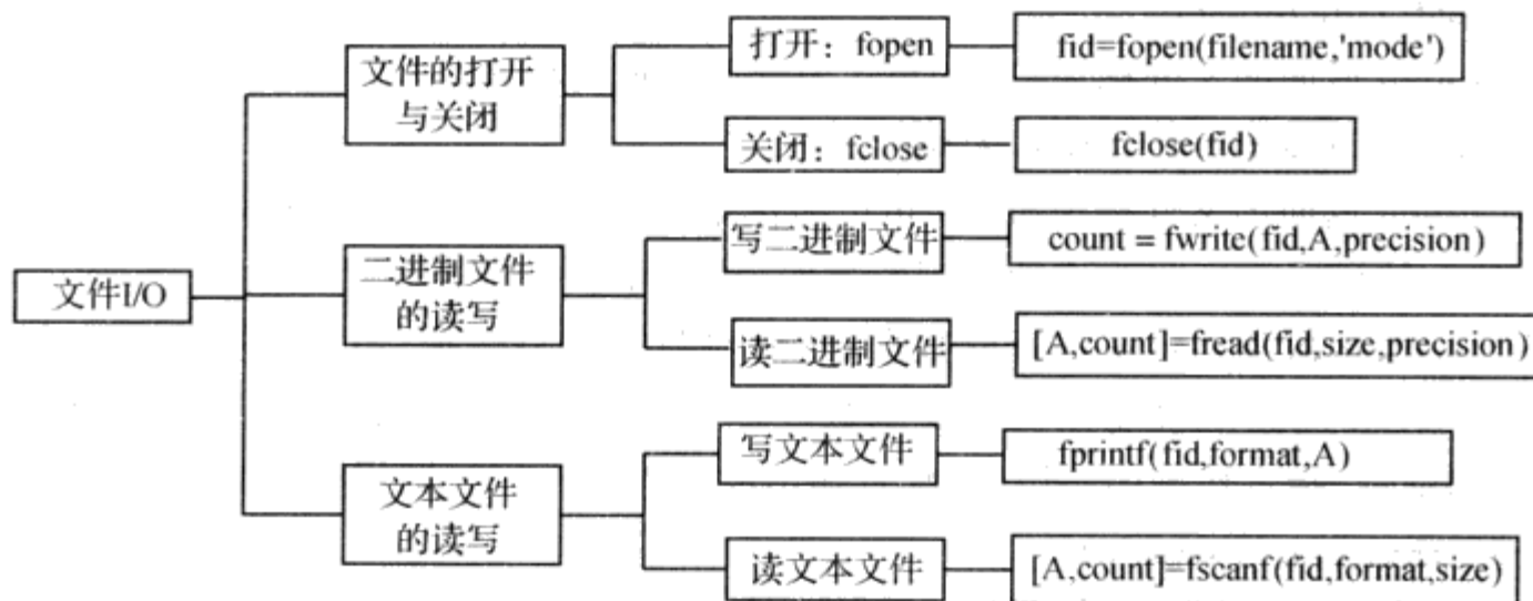
图 2.12 低级文件 I/O 操作框图
