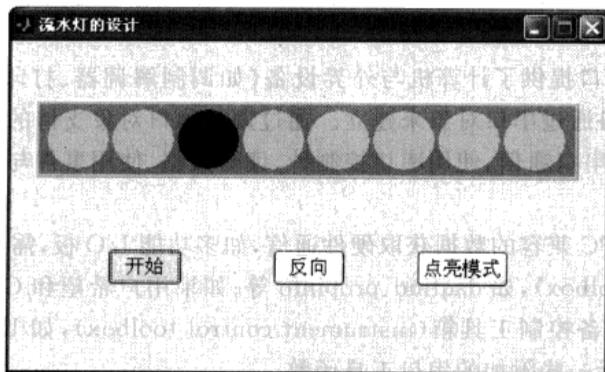
图 8.12 例 8.4.4 运行结果
