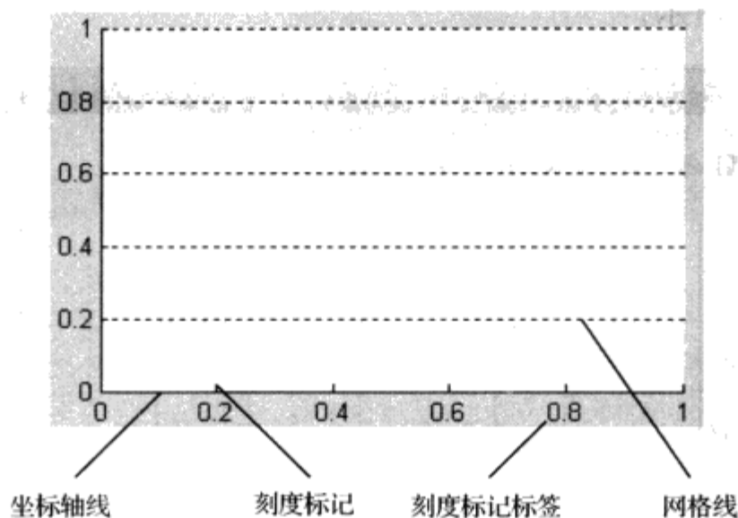
图 4.9 坐标线
