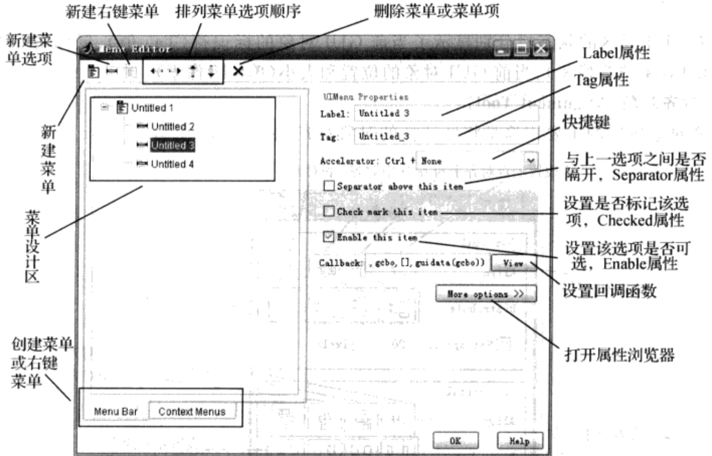
图 6.11 菜单编辑器
