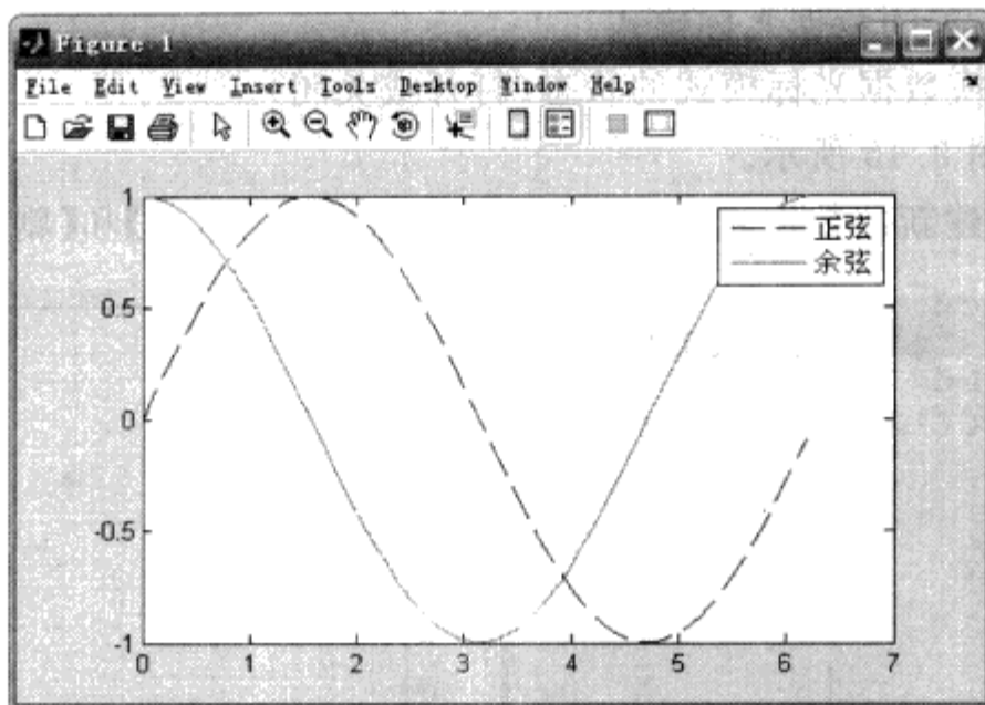
图 3.16 显示图例
