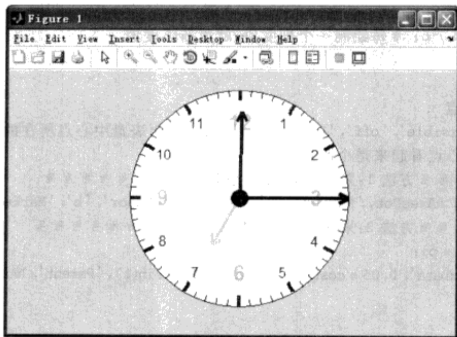
图 4.84 例 4.3.3 效果图
