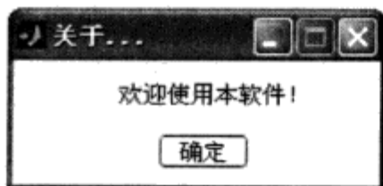
图 5.16 普通对话框
