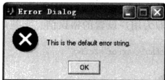
图 5.17 错误对话框
