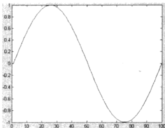
图 3.1 plot(sin(t)) 结果
