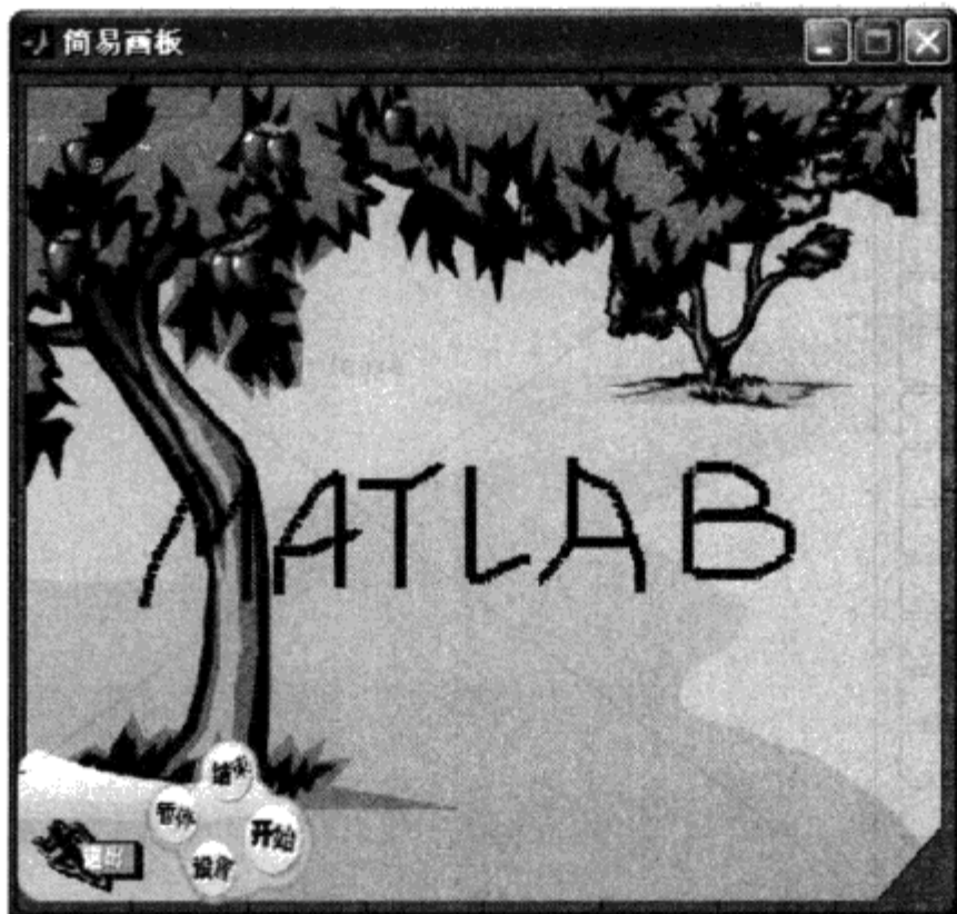
图 6.56 例 6.3.3 运行结果
