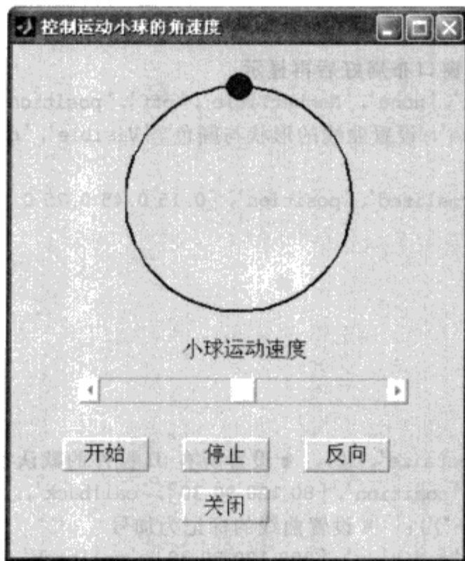
图 4.88 例 4.4.2 原图
