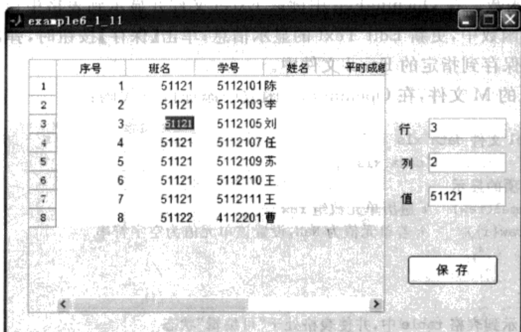
图 6.50 例 6.1.11 运行结果
