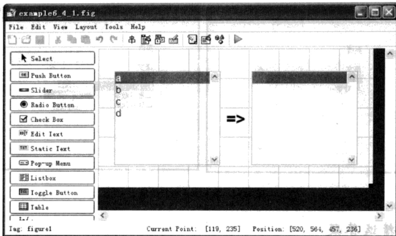
图 6.64 例 6.4.1 界面设计
