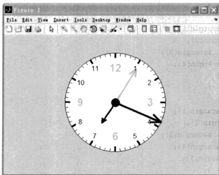
图 4.85 例 4.3.4 效果图
