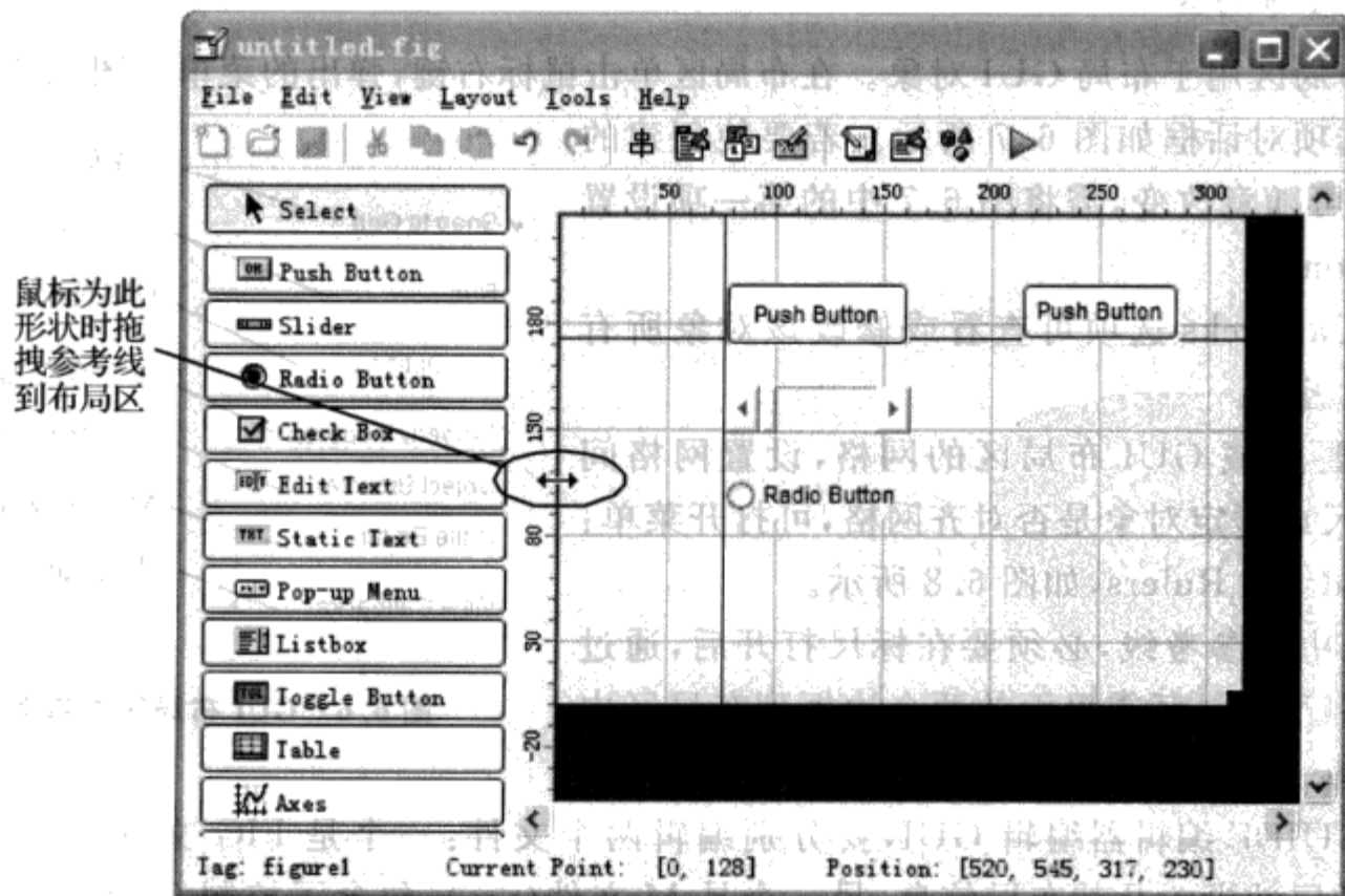
图 6.9 创建参考线
