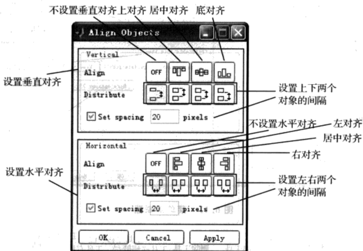
图 6.10 对齐对象
