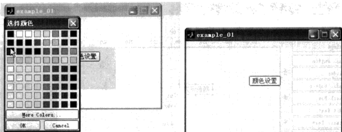
图 6.30 例 6.1.1 运行结果
