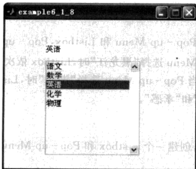
图 6.43 例 6.1.8 运行结果
