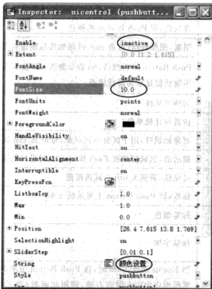
图 6.27 属性设置
