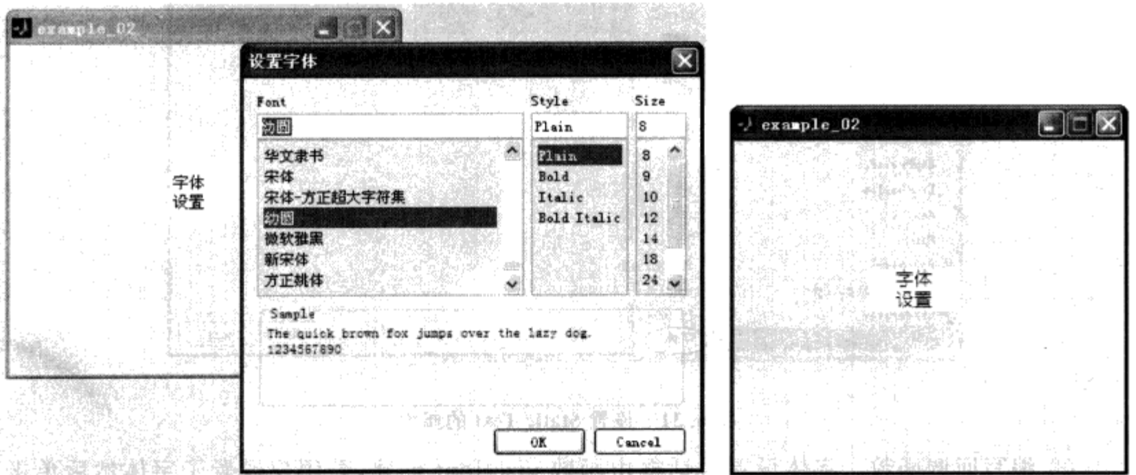
图 6.33 例 6.1.2 运行结果
