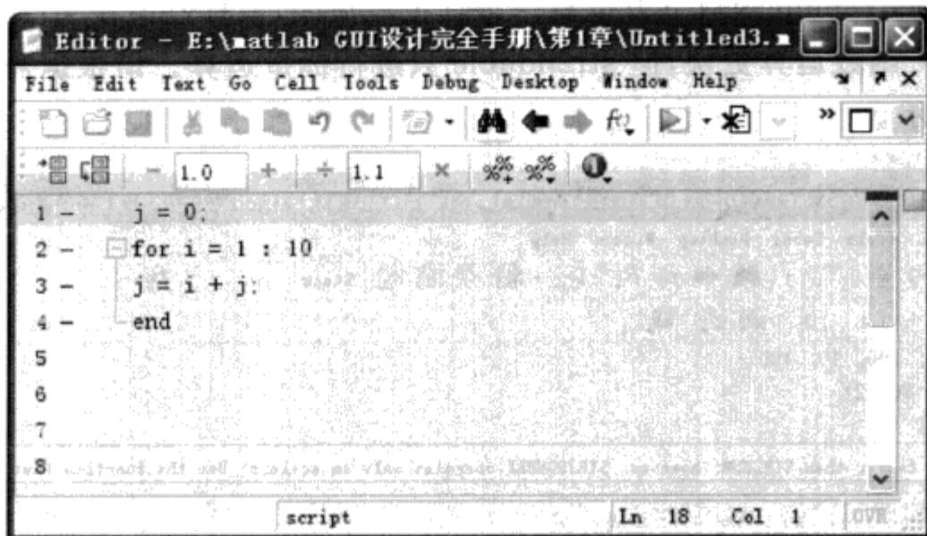
图 1.25 未缩排的代码
