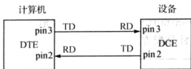
图 9.2 DTE 与 DCE 之间的连接
