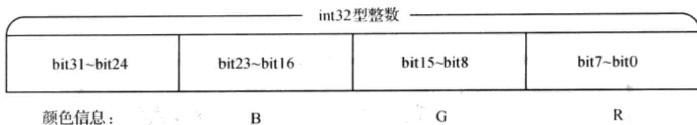
图 7.9 BackColor 值的存储格式
