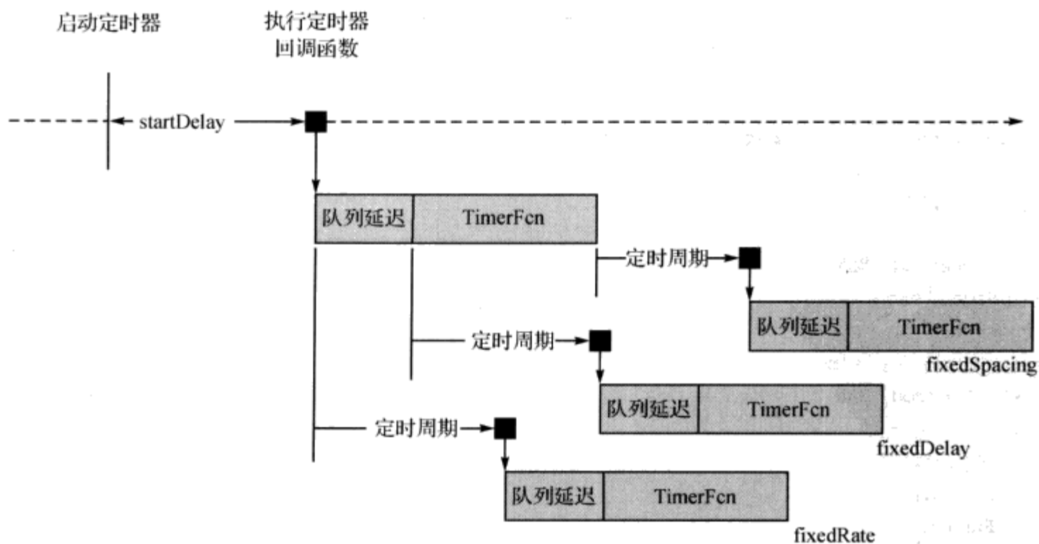
图 8.2 fixedRate、fixedDelay 和 fixedSpacing 模式
